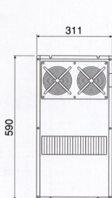
● 外形図
