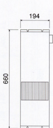
● 外形図
