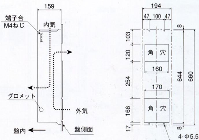
● 取付穴寸法図
