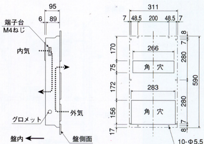
● 取付穴寸法図
