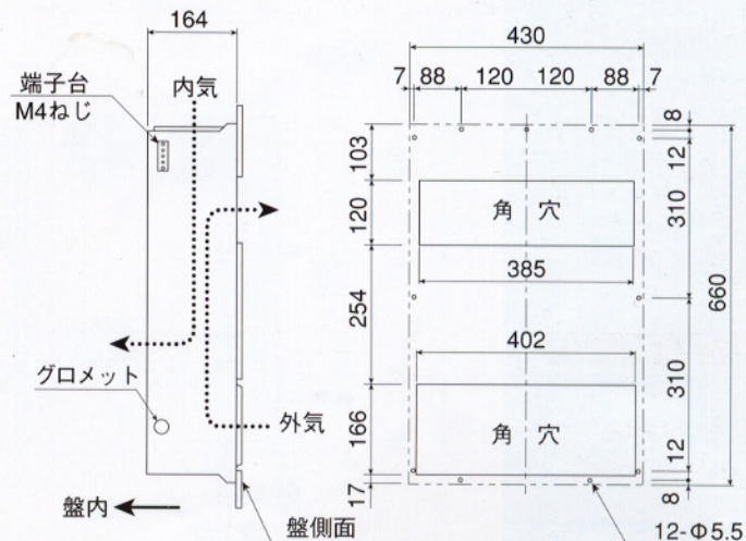
● 取付穴寸法図
